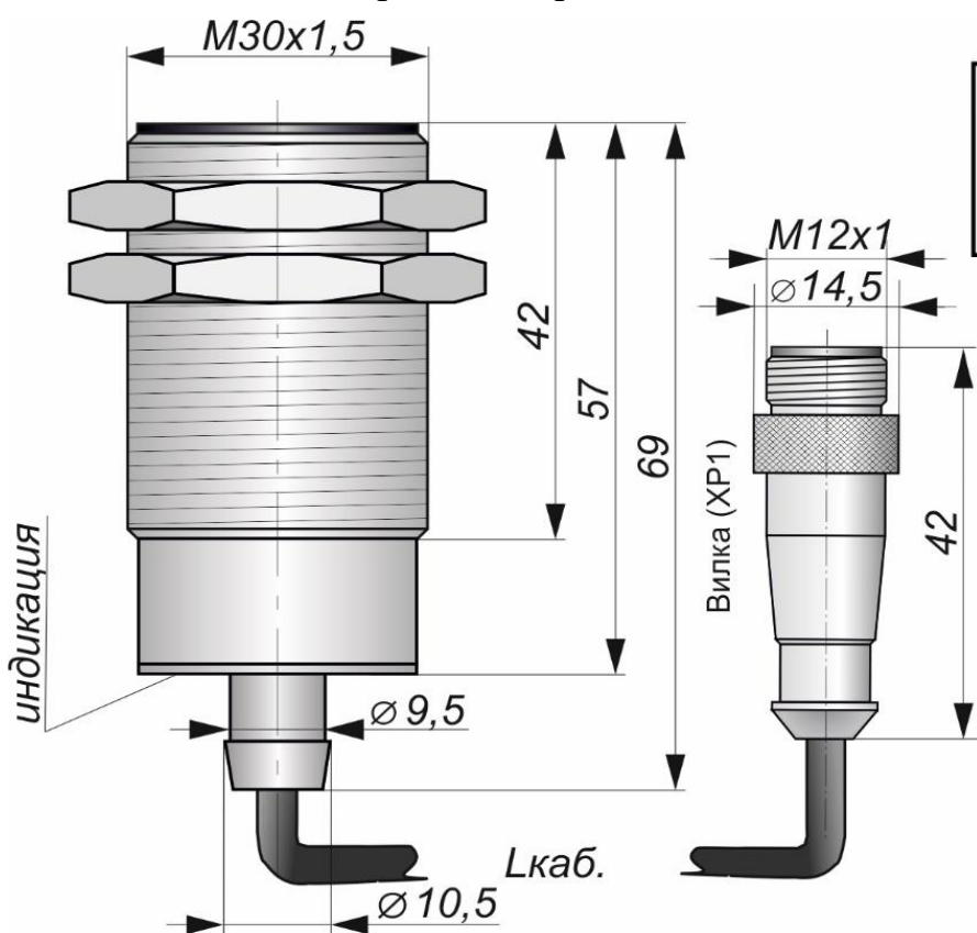
Габаритный чертеж
